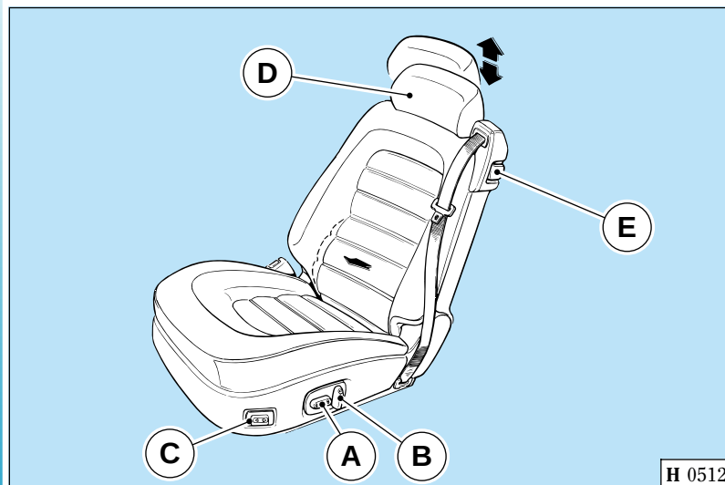
Fig. 15 - Sedili elettrici.
