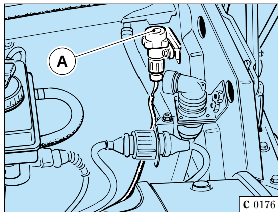
Fig. 3 - Interruttore inerziale.
