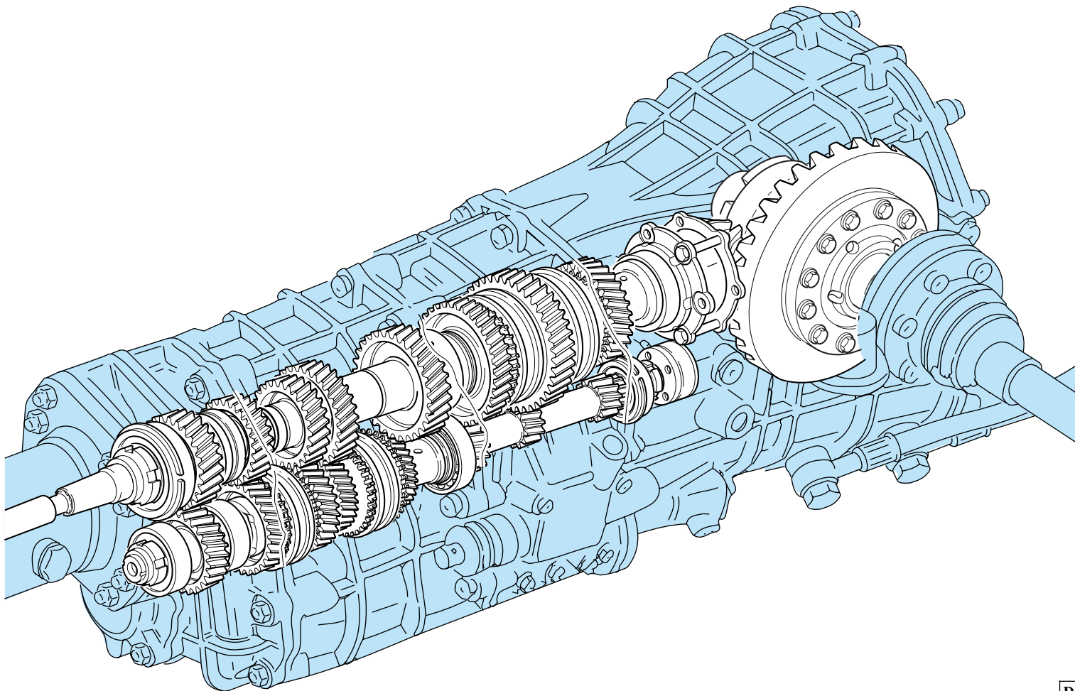
Fig. 9 - Cambio e differenziale.
