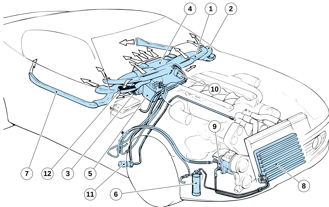
Fig. 1 - Impianto climatizzazione
