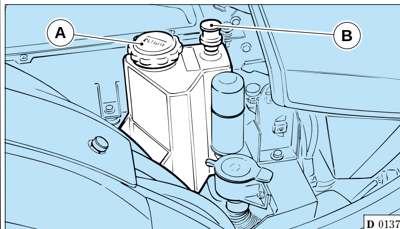
Fig. 3 - Serbatoio olio per idroguida
