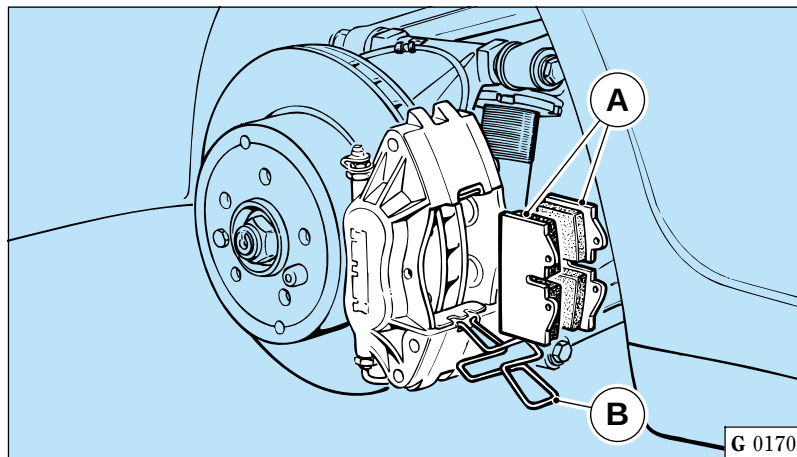
Fig. 6 - Sostituzione pastiglie freno posteriori
