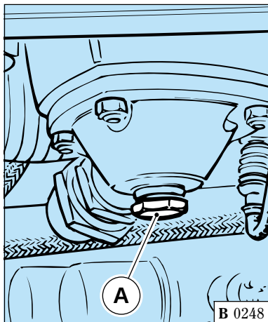
Fig. 6 - Sostituzione olio
