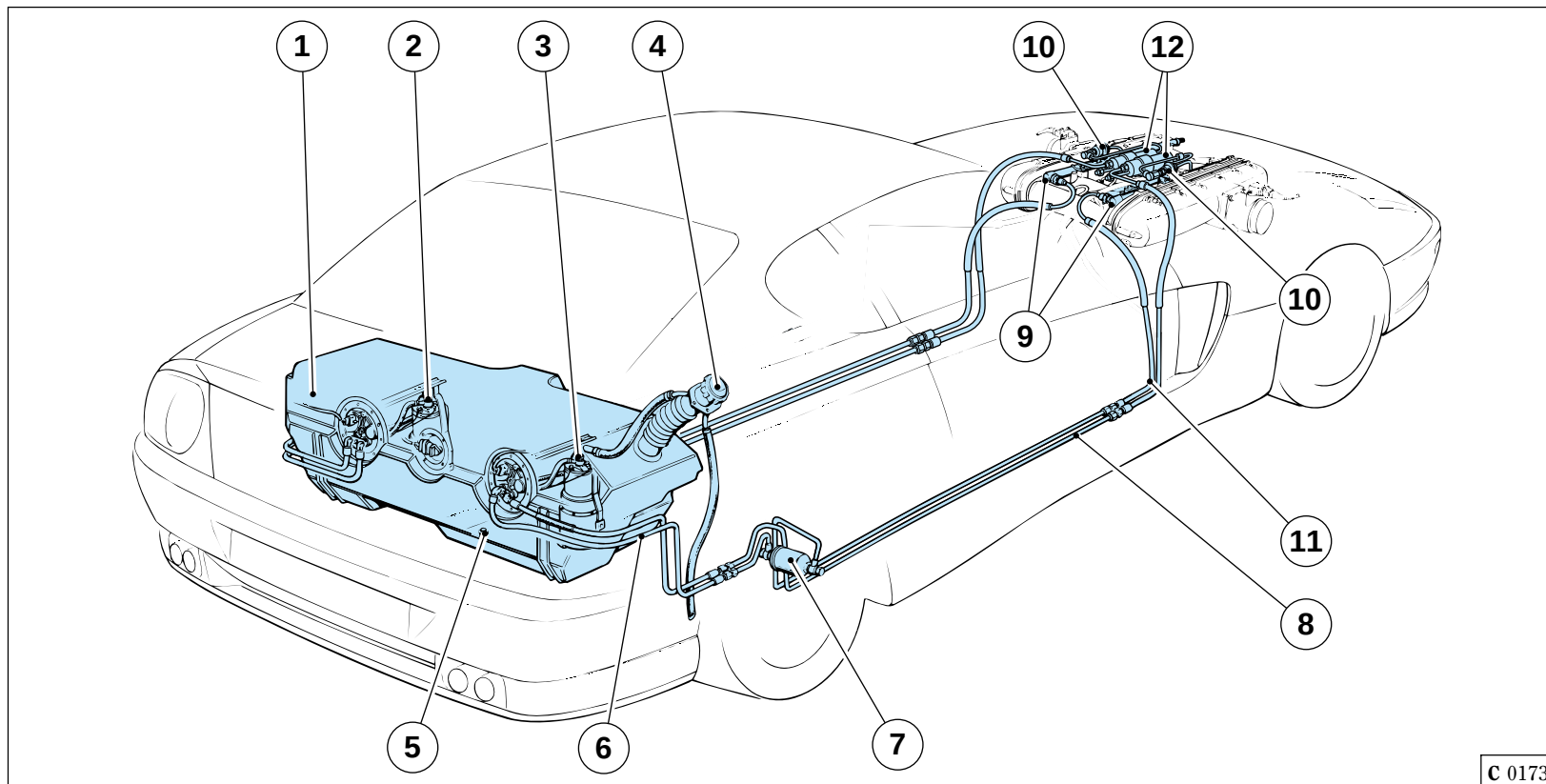
Fig. 2 - Impianto alimentazione carburante 1 - Serbatoio carburante; 2 - Pompa benzina Sx; 3 - Pompa benzina Dx; 4 - Bocchettone di carico; 5 - Tappo scarico carburante; 6 - Tubazione di mandata benzina; 7 - Filtro benzina; 8 - Tubazione di mandata benzina; 9 - Collettore con iniettori; 10 - Regolatore pressione carburante; 11 - Tubazioni ritorno benzina; 12 - Scambiatore di calore freon/benzina.
