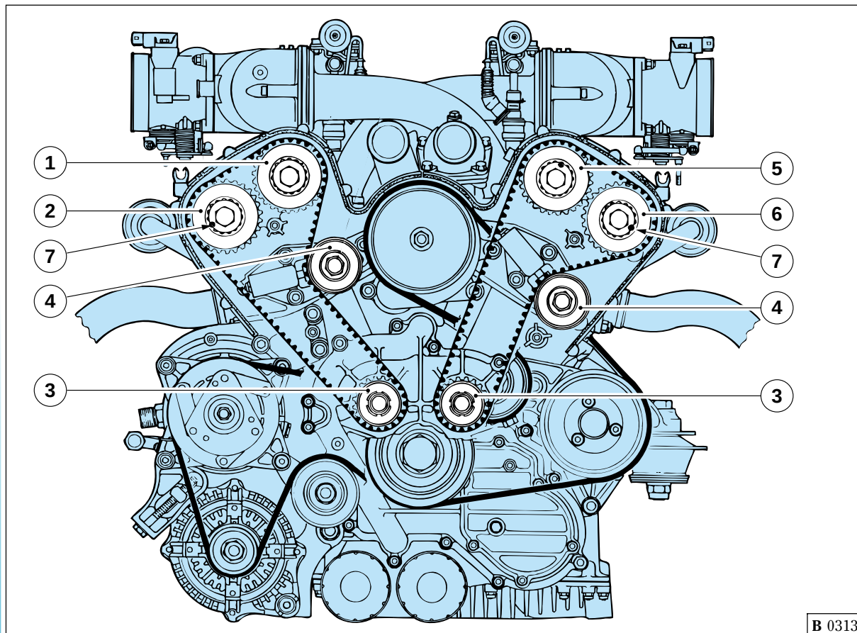
Fig. 2 - Schema comando distribuzione
