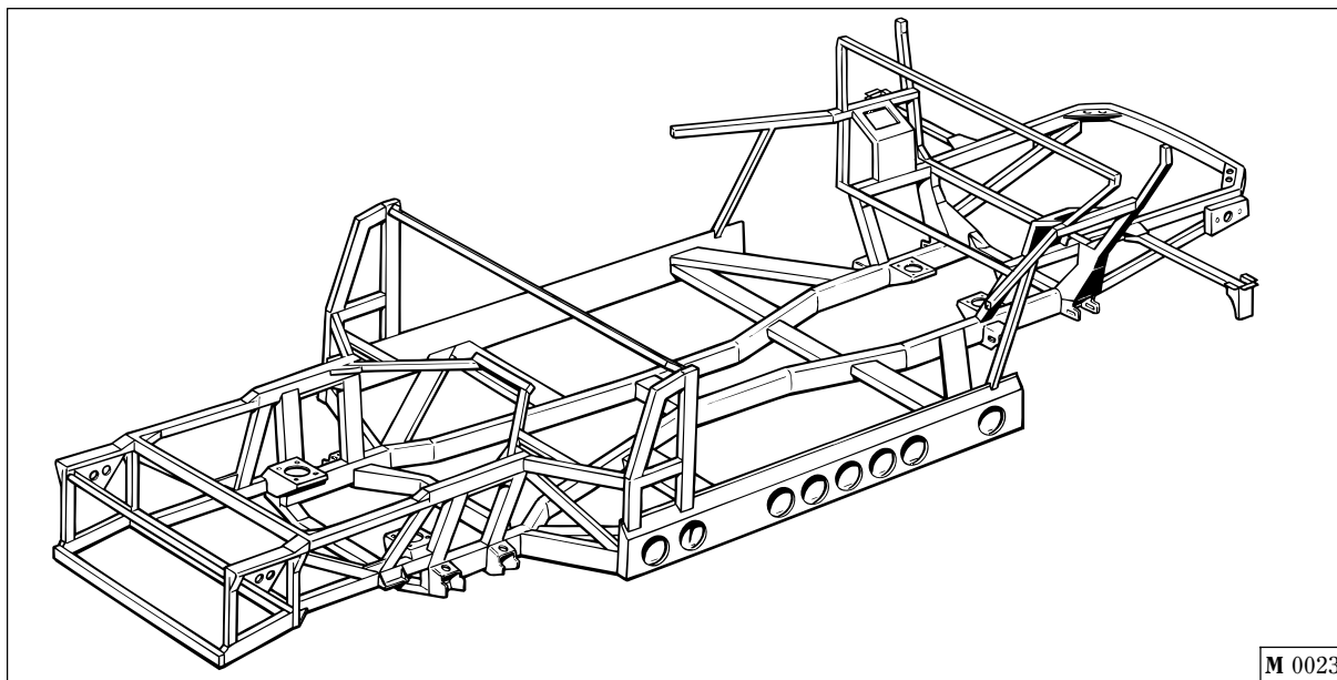
Fig. 1 - Telaio.
