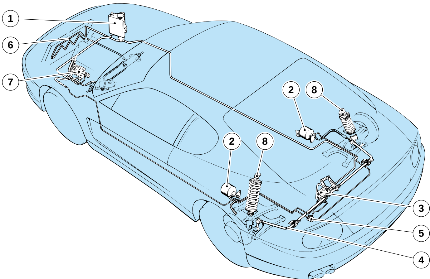
Fig. 5 - Schema impianto controllo altezza assale posteriore
