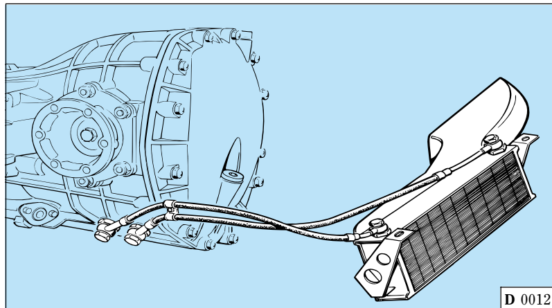
Fig. 11 - Circuito di raffreddamento.
